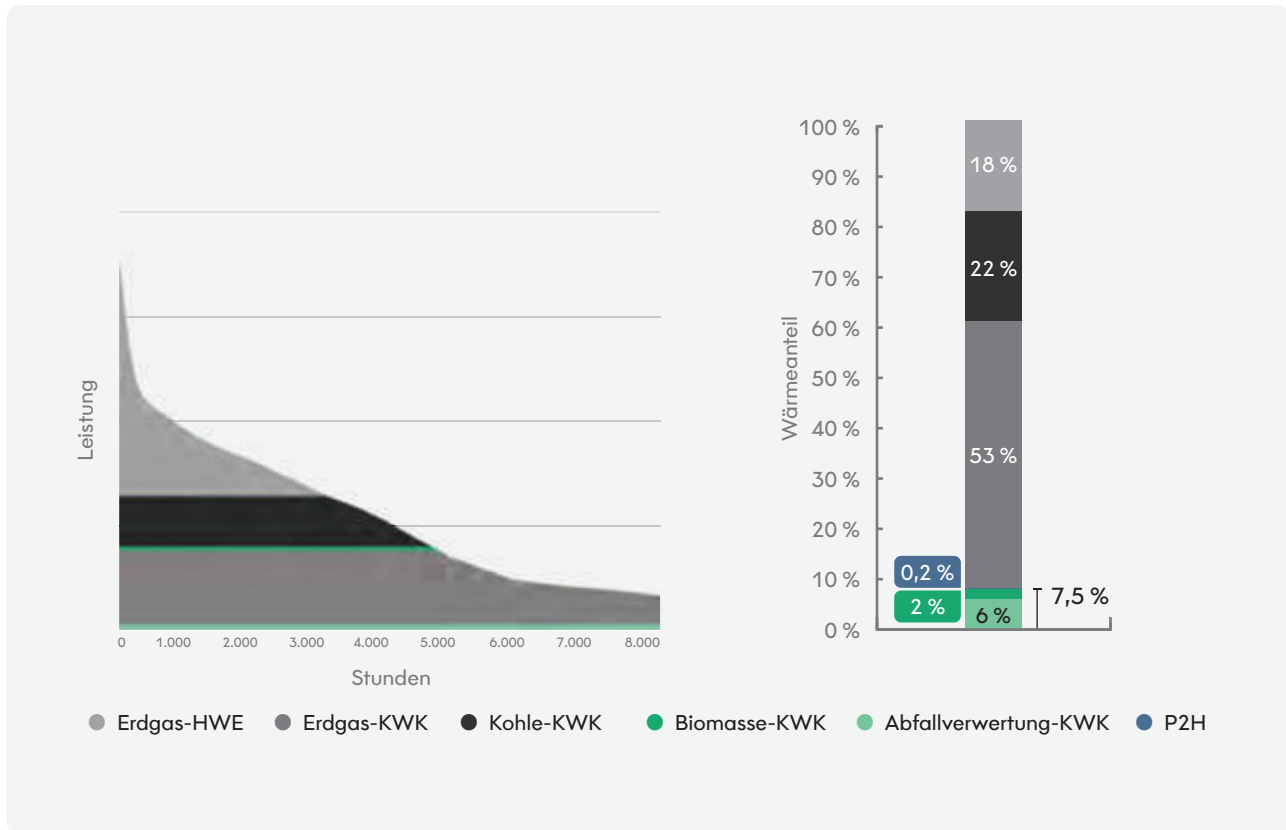
Abbildung 6: Schematischer Anlageneinsatz im Verbundnetz 2024
