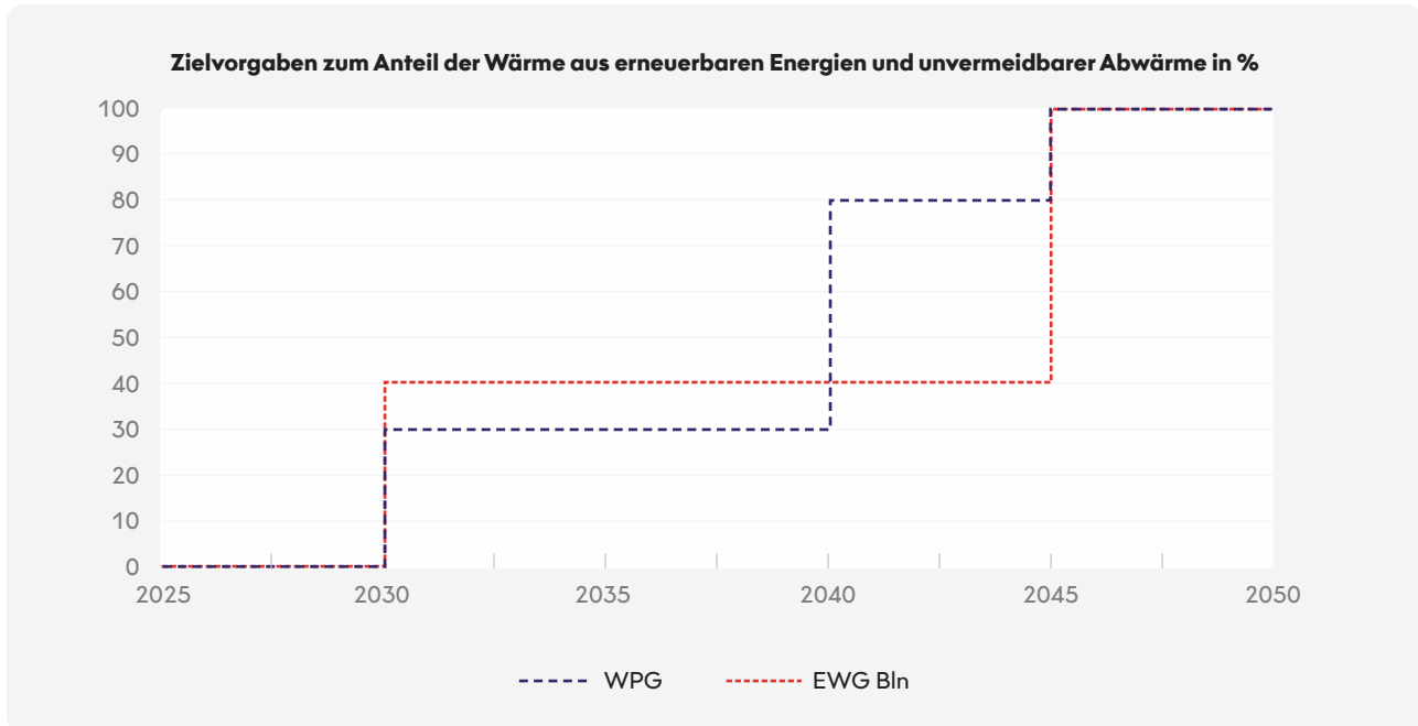
Abbildung 7: Mindestanteile erneuerbarer Energien und/oder unvermeidbarer Abwärme
